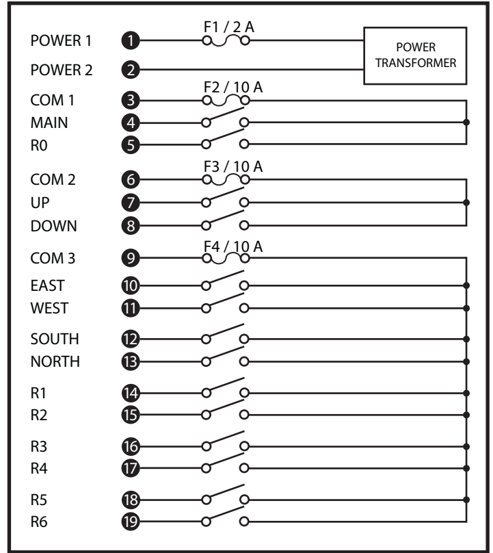
Q1200 Wiring diagram
