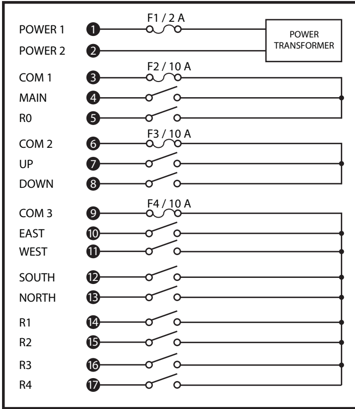
Q1010 Wiring diagram
