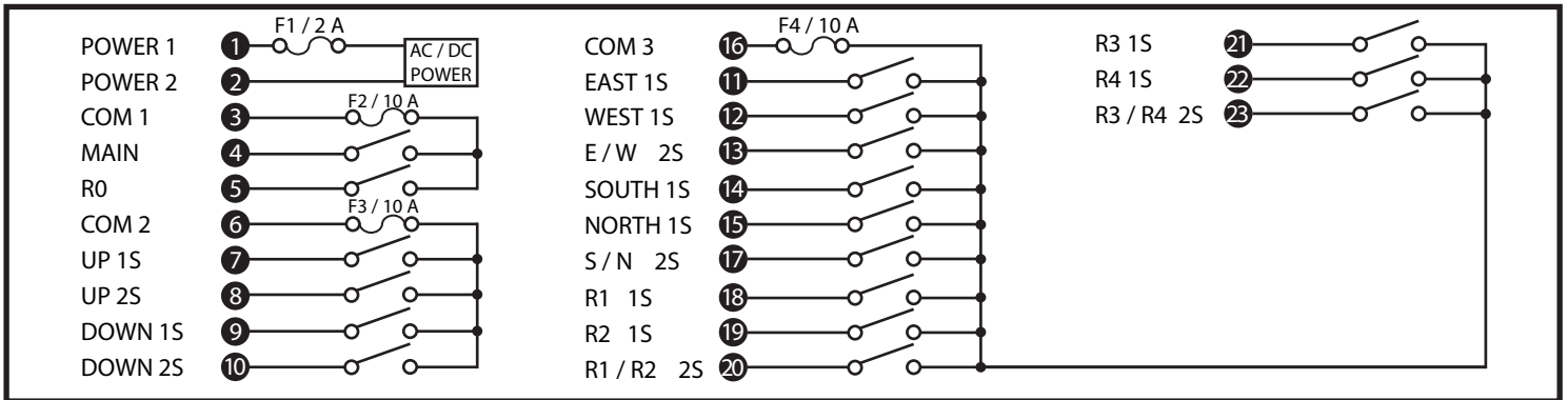
Q1212 Wiring diagram
